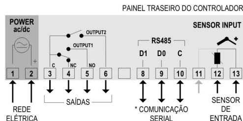
Fig. 1 – Conexões mostradas na etiqueta do controlador
